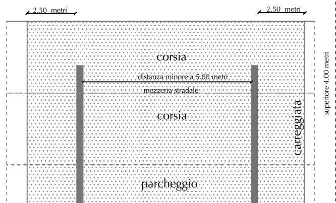
figura 29 duplici attraversamenti del parcheggio e della carreggiata
