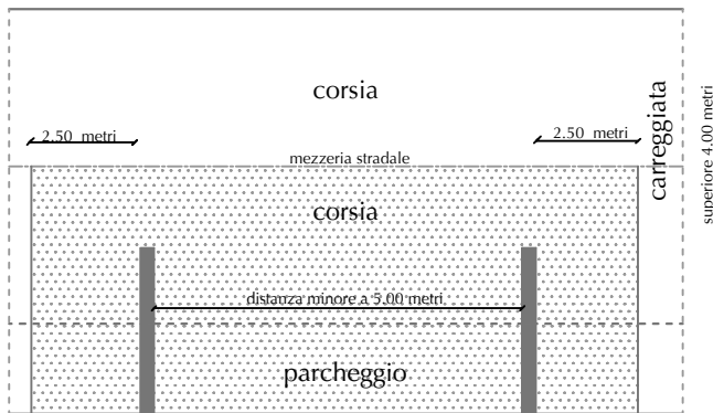
figura 26 attraversamento del parcheggio e della carreggiata
