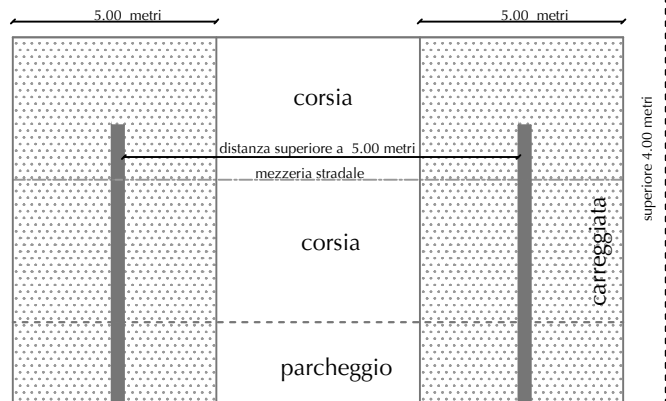
figura 28 duplici attraversamenti del parcheggio e della carreggiata
