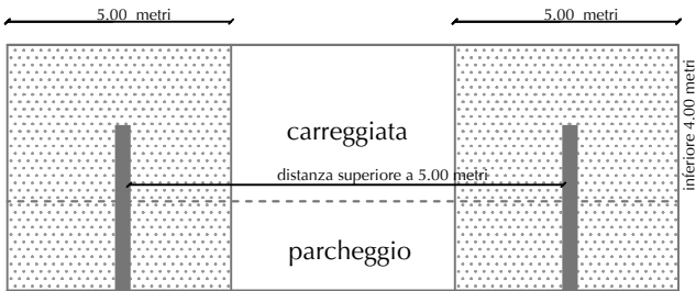
figura 22 attraversamenti multipli del parcheggio e della carreggiata
