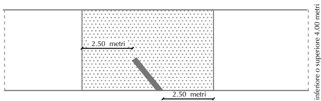
figura 32 attraversamento della strada
