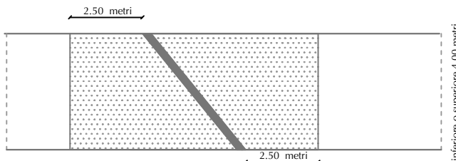
figura 33 attraversamento della strada
