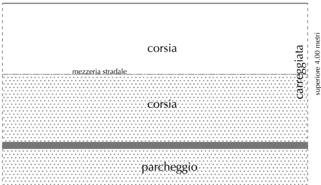
figura 31 scavo longitudinale tra parcheggio e carreggiata
